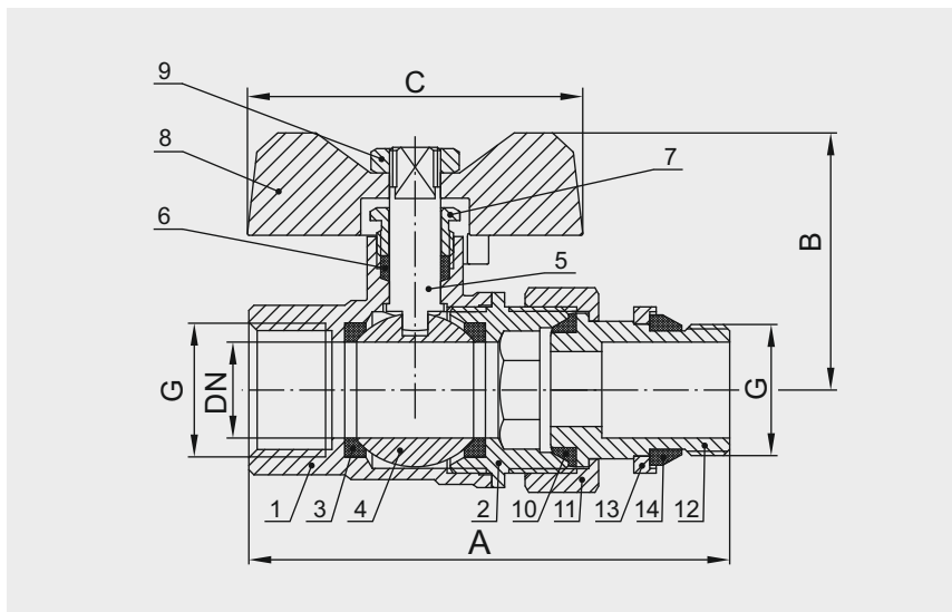
Кран с полусгоном и кольцевым уплотнением, прямой PF UBV 324UR – PF UBV 326UR
