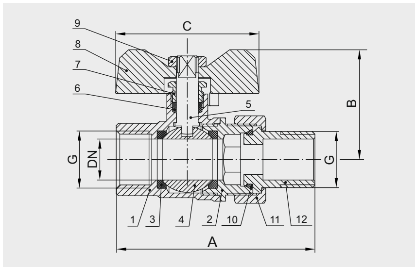
Кран с полусгоном, прямой PF UBV 324S – 327S
